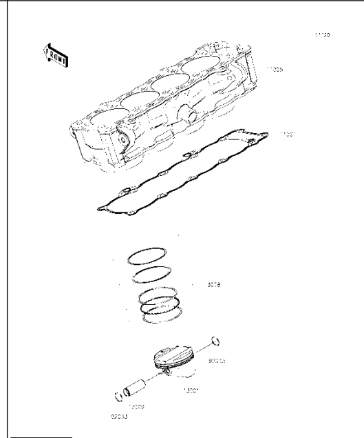
K3 Cylinder/Piston(s)
